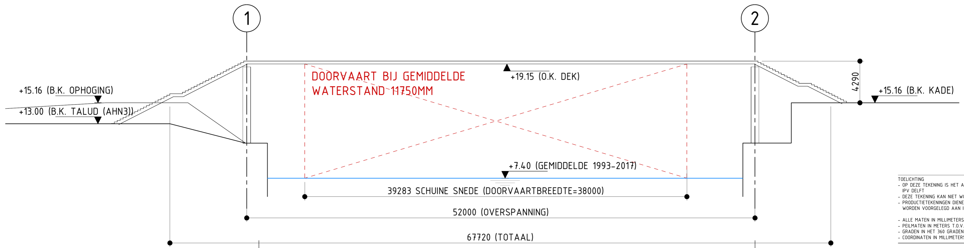
PROFIEL: WATERSTAND GEMIDDELD TUSSEN 1993-2017 (221 DAGEN TOEGANKELIJK) SCHAAL 1:200
