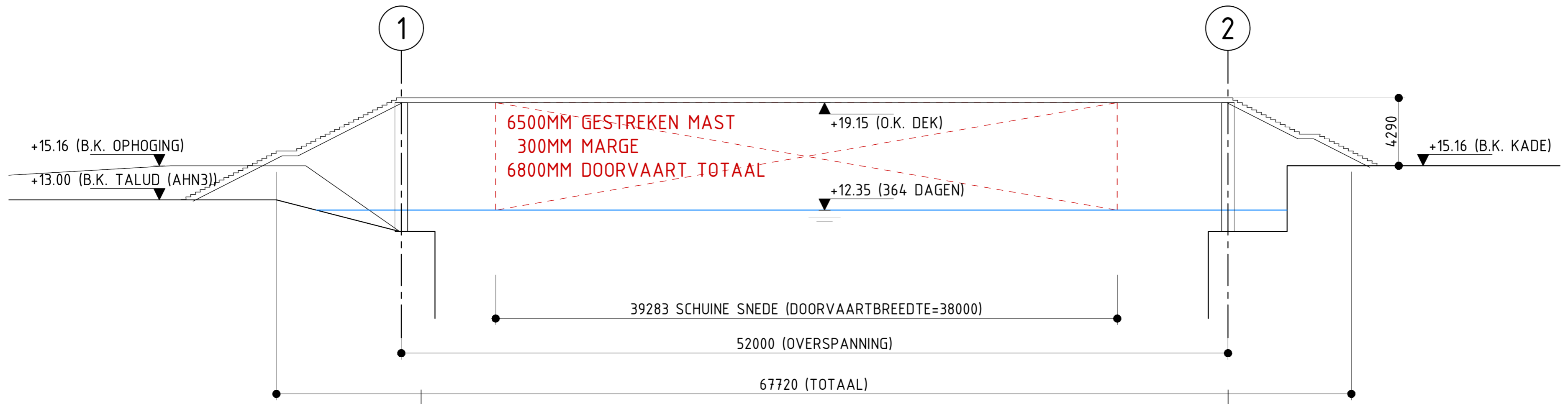
PROFIEL: WATERSTAND HOOG (364 DAGEN TOEGANKELIJK) SCHAAL 1:200
