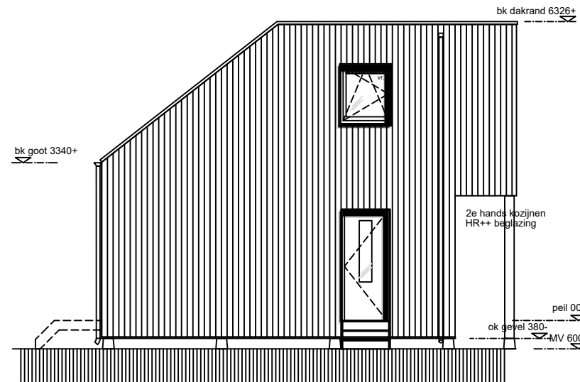
Gevel west
