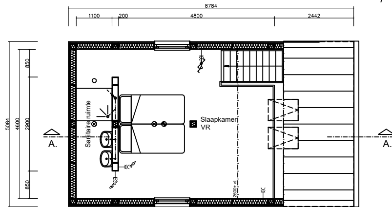
1e verdieping
