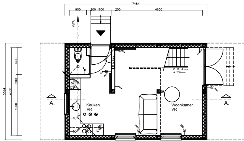
Begane grond
