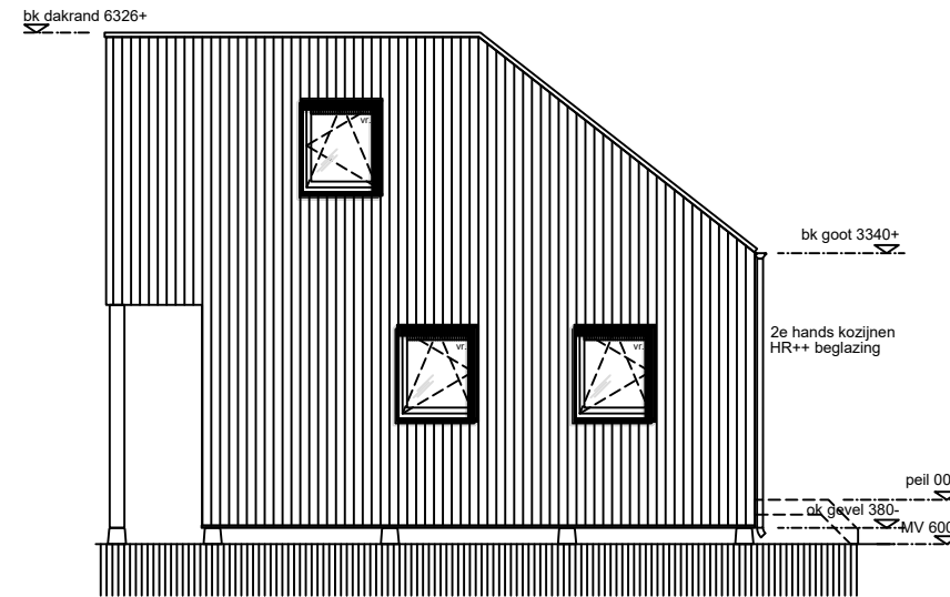
Gevel oost
