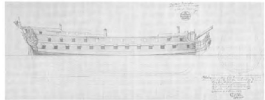
Linjeskeppet Prinsessan Sophia Albertina. Ritning av G. Sheldon 1759, Sjöhistoriska Museet. Foto: Johan Johnson
